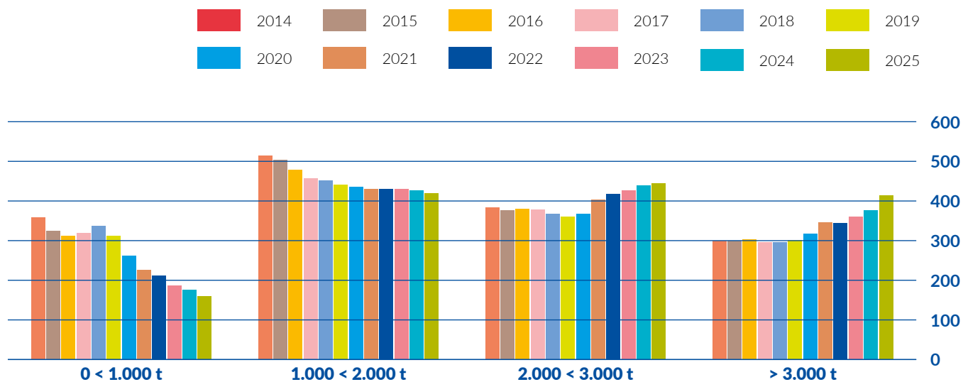
AFBEELDING 10: TANKVLOOT IN DE RIJNOEVERSTATEN NAAR LAADVERMOGEN
