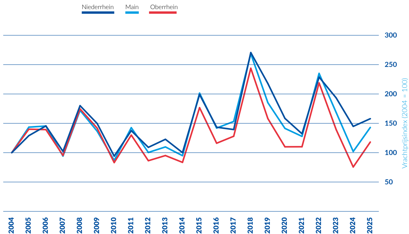
AFBEELDING 5: INSIGHTS GLOBAL-VRACHTPRIJSINDEX VOOR HET VERVOER VAN VLOEIBARE LADING (GASOLIE) IN HET ARA-RIJNSTROOMGEBIED (2004 = 100), GECORRIGEERD VOOR DE GESTEGEN KOSTEN
